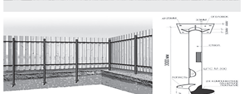
Устройство ограждения мусульманского кладбища д. Сосновка
