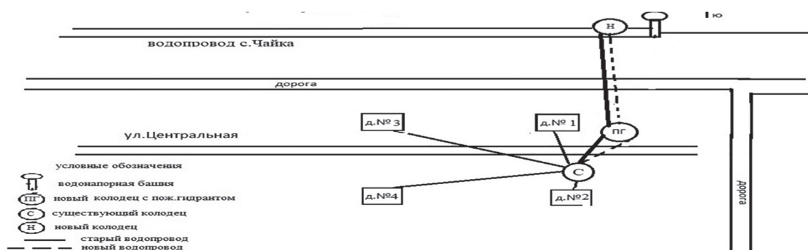
Схема текущего ремонта водопроводных сетей в с. Суда по ул. Центральная от дома № 1 до дома № 6
